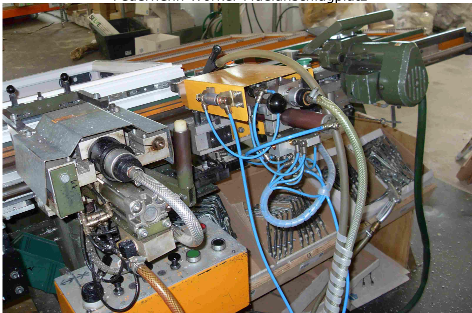
Bearbeitungsaggregate: Schrauben, Bohren, Olivenbohren Schlosskastenfräsen
