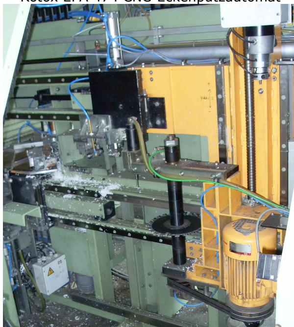
Bearbeitungsaggregate EPA 474
